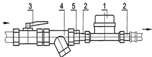
Рисунок 1 - Варианты подключения Счетчика
