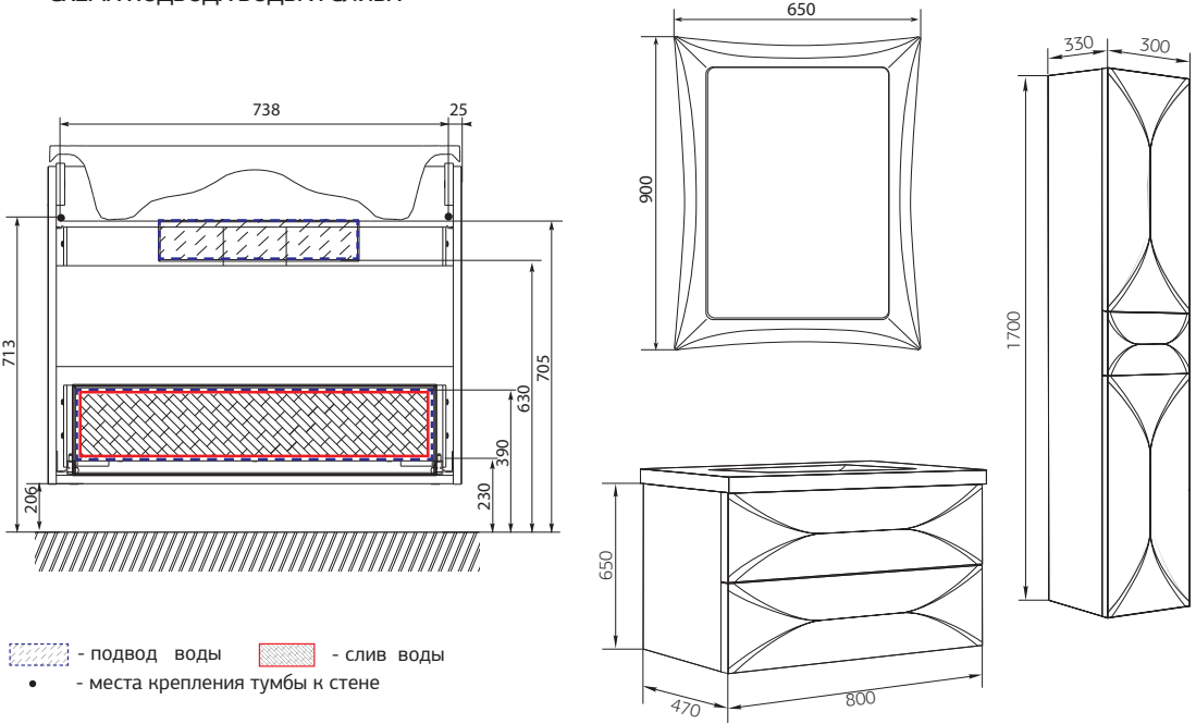
СХЕМА ПОДВОДА ВОДЫ И СЛИВА
