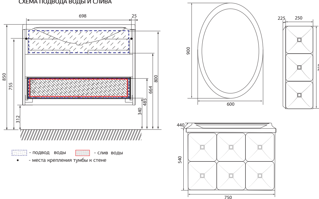
СХЕМА ПОДВОДА ВОДЫ И СЛИВА
