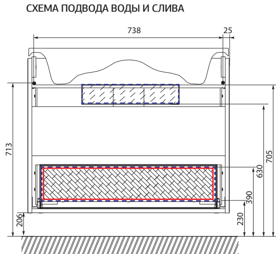
СХЕМА ПОДВОДА ВОДЫ И СЛИВА
