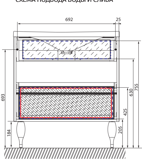
СХЕМА ПОДВОДА ВОДЫ И СЛИВА
