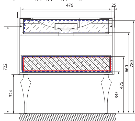
СХЕМА ПОДВОДА ВОДЫ И СЛИВА
