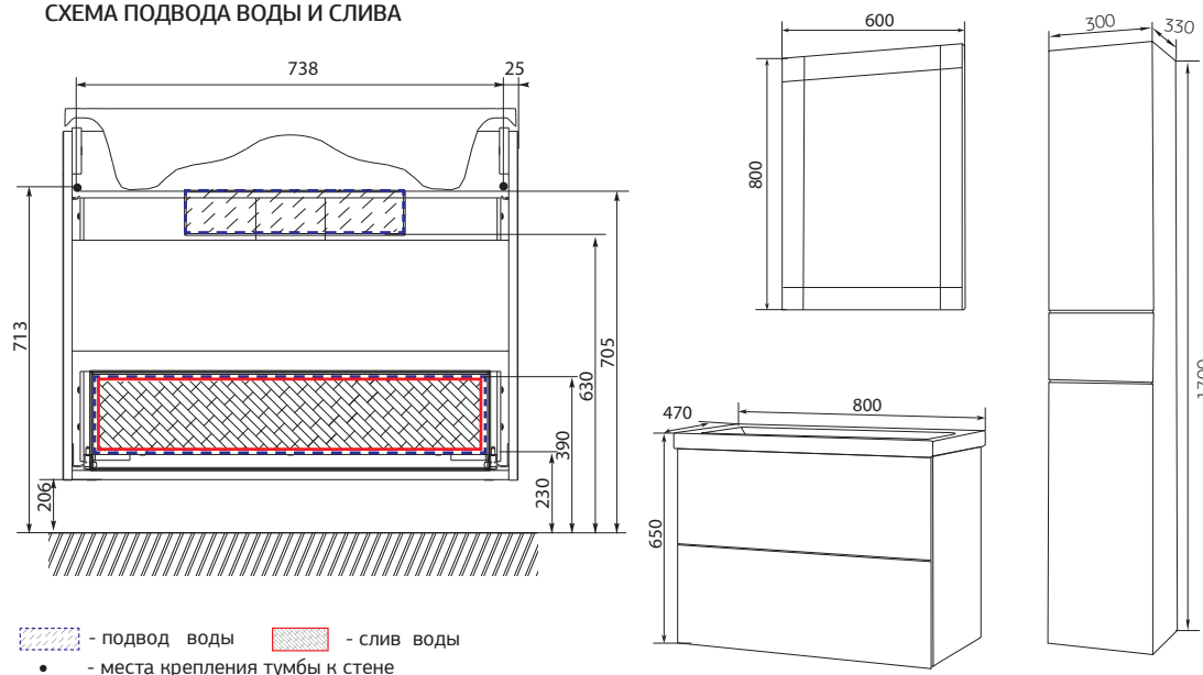
СХЕМА ПОДВОДА ВОДЫ И СЛИВА
