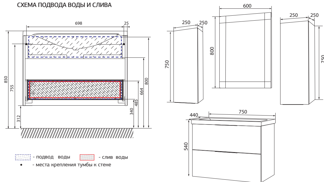
СХЕМА ПОДВОДА ВОДЫ И СЛИВА
