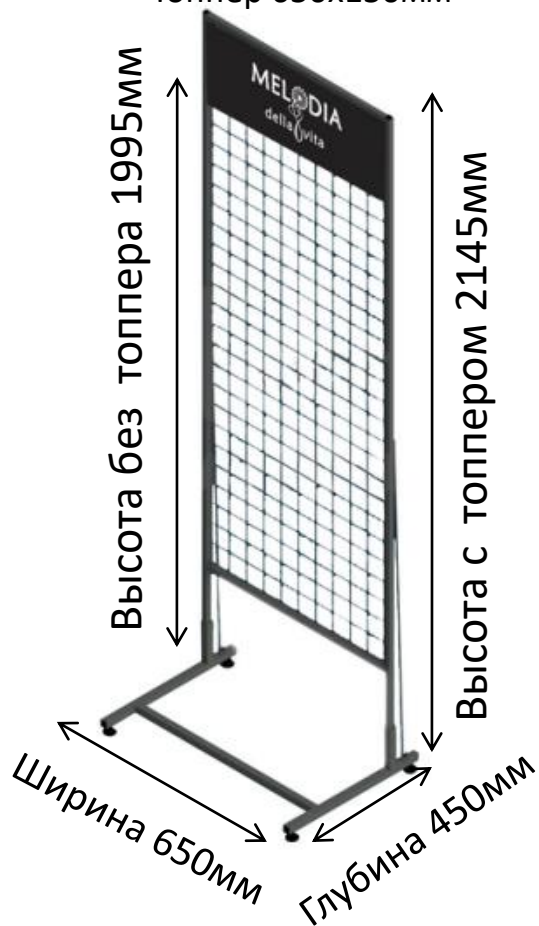
Стенд пристенный 650x450мм
