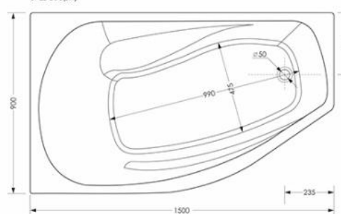
Акриловая ванна Jazz левая Вид сверху
