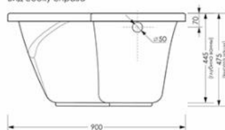
Акриловая ванна Jazz левая Вид сбоку справа
